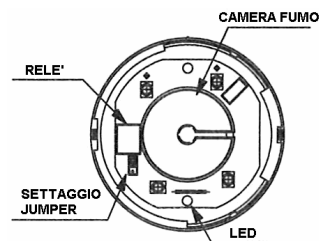
Fig. 3 Schema del rivelatore con coperchio rimosso
